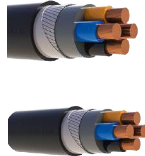
XLPE İzoleli Yassı Çelik Tel Zirhli Alçak Enerji Kabloları
