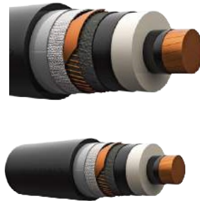
Suya Dayanıklı Orta Gerilim Kabloları
